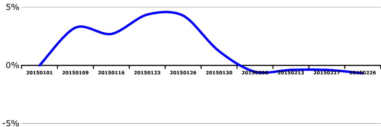
达摩掌 2015 年的累积收益曲线 (激进型)
