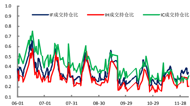
图 8 期货主力合约成交持仓比
