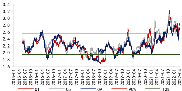
图9 油粕比
