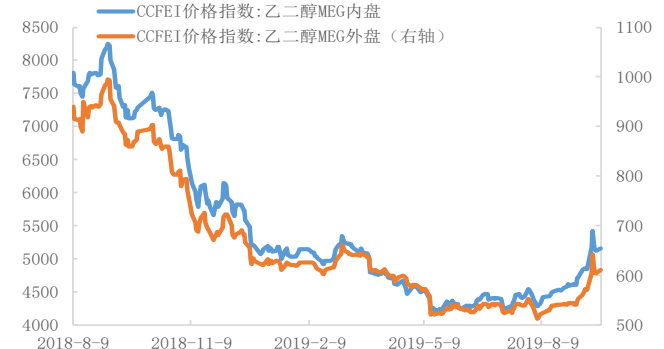
图 6 MEG 价格
