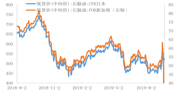
图 4 石脑油价格
