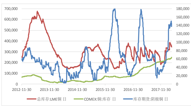
图 5 铜库存
